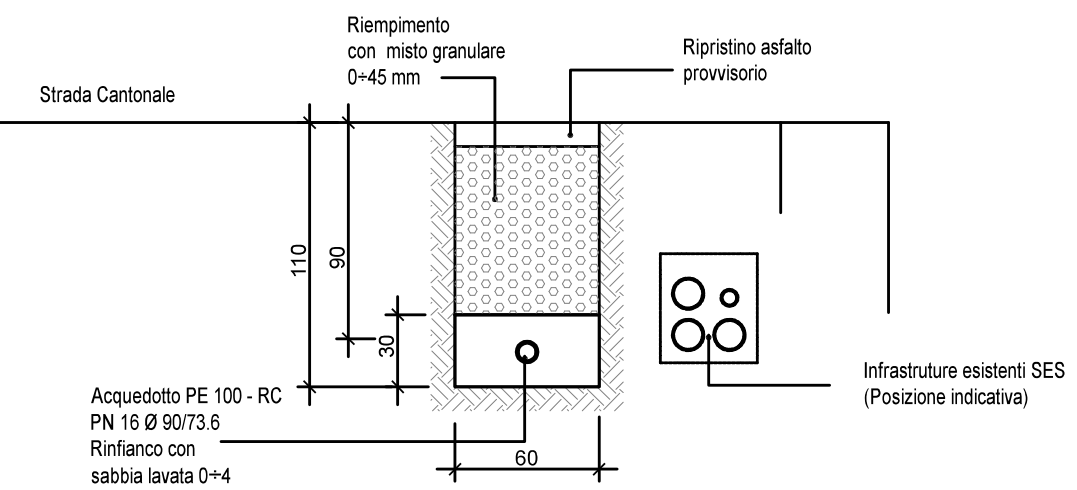
Sezione tipo 1 - 1:25
