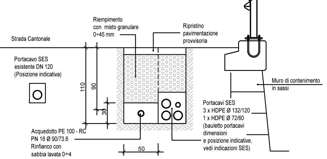
Sezione tipo 2 - 1:25
